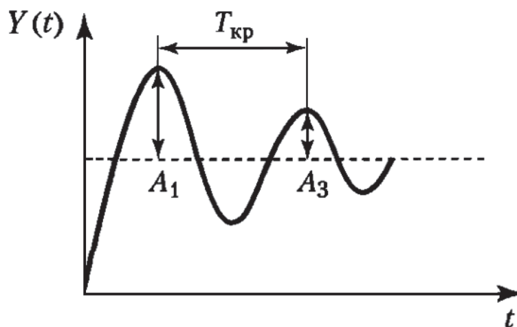
Рисунок 7.4 – Форма сигнала в методе затухающих колебаний
