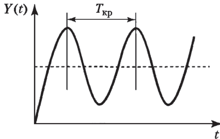
Рисунок 7.3 – Форма сигнала в методе незатухающих колебаний
