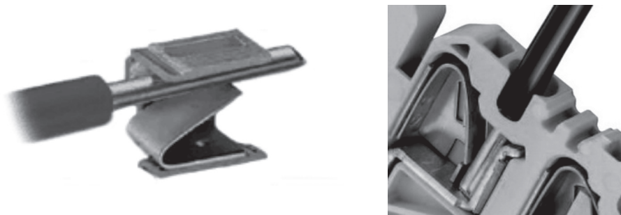
Рисунок 6.13 – Штекерный зажим
