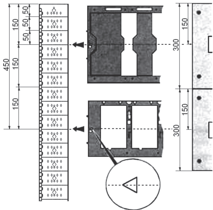
Рисунок 6.6 – Регулируемые крепежные элементы и пластины
