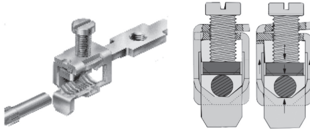
Рисунок 6.9 – Винтовая клемма
