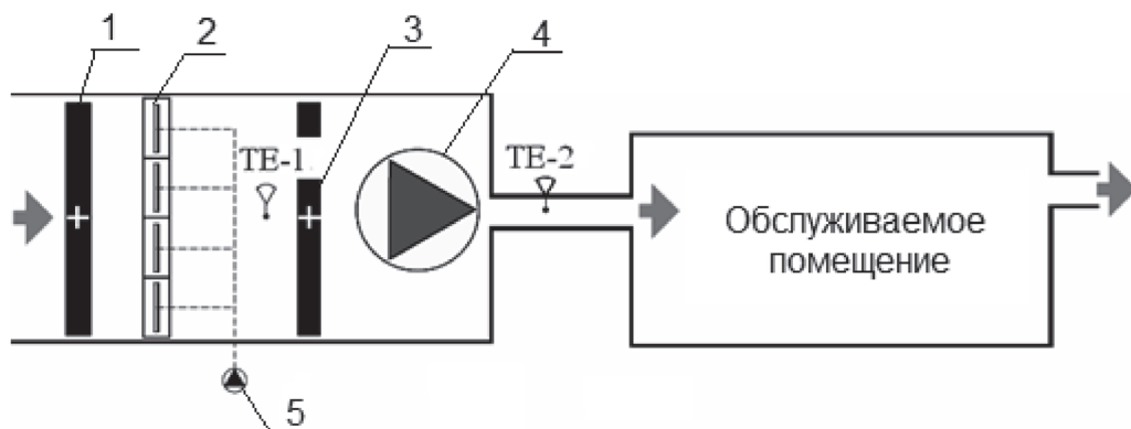
1 – первый нагреватель; 2 – кассеты увлажнителя; 3 – второй нагреватель; 4 – вентилятор; 5 – насос; ТЕ-1 – датчик точки росы; ТЕ-2 – датчик температуры
