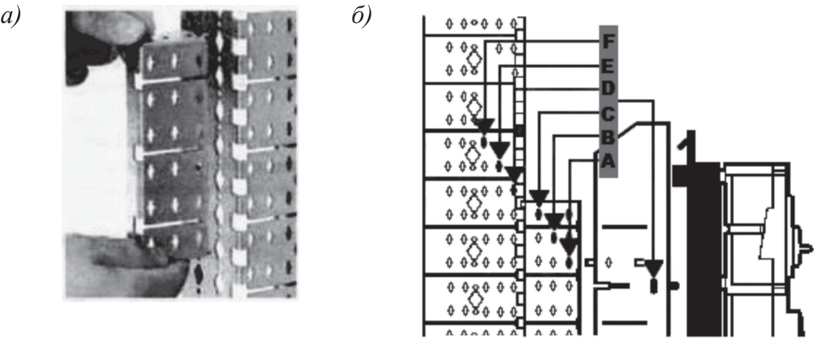
а) крепление регулятора глубины на монтажной стойке; б) шесть положений размещения аппаратуры по глубине электроконструкции, обозначаемые буквами от А до F
