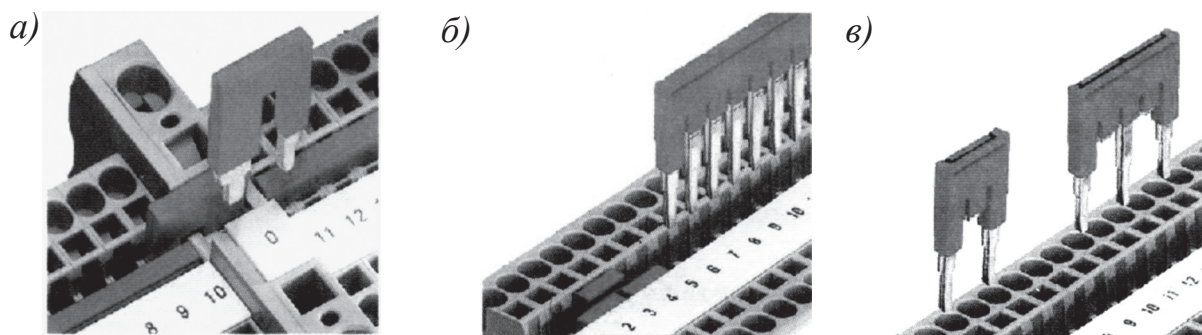
а) маркировка; б) шунтирование штекерными перемычками; в) шунтирование перемычками с пропусками
