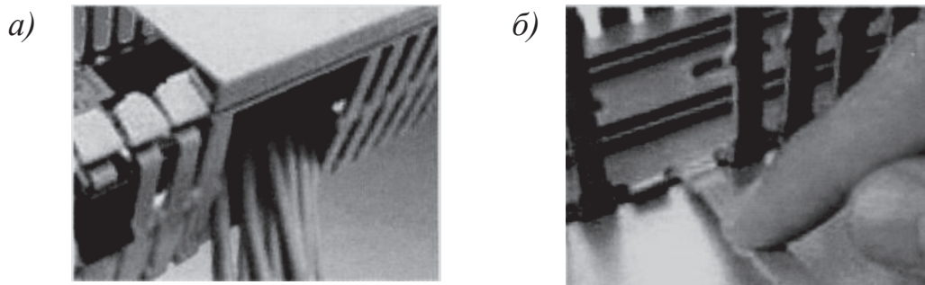
а) вывод из канала проводов; б) выламывание боковых гребенок
