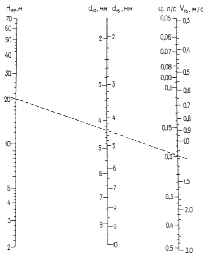
Черт.6. Номограмма для определения диаметров отверстий диафрагм, устанавливаемых у смесителей водоразборной арматуры санитарных приборов d_{10} ( d_{15} ) - диаметр отверстия диафрагмы, мм, устанавливаемой в соединительных патрубках (подводках) смесительной водоразборной арматуры с условным проходом d' = 10 и 15 мм; v_{15} - скорость движения воды, м/с, в подводке d' = 15 мм
