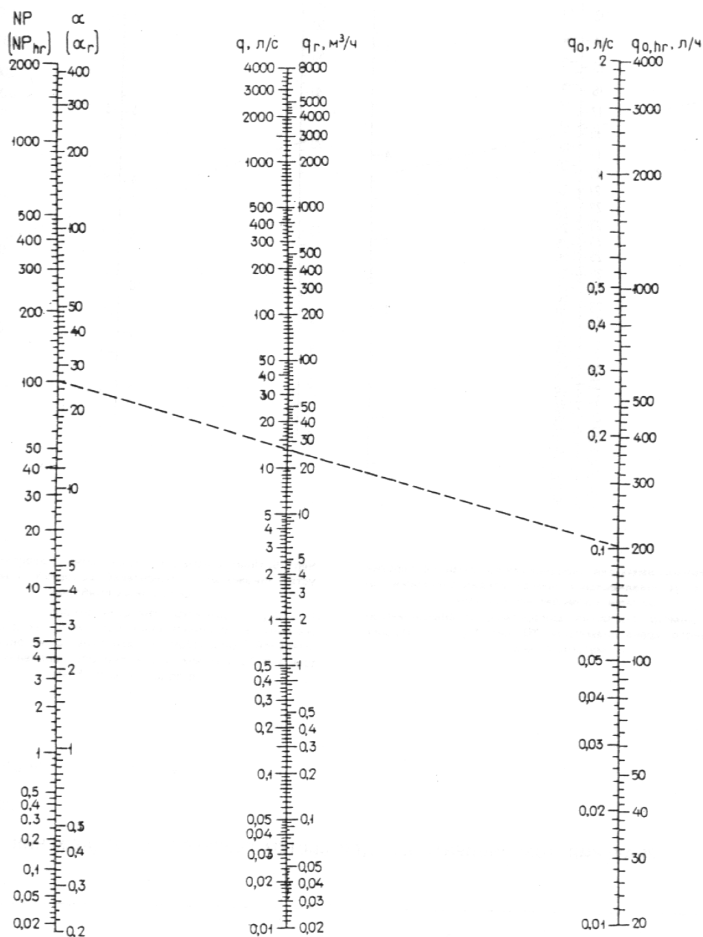
Черт.4. Номограмма для определения секундных и часовых расходов воды в зависимости от NP ( NP_{hr} ) при различных значениях q_0, \text{л/с} , q_0, \text{hr, л/ч}
