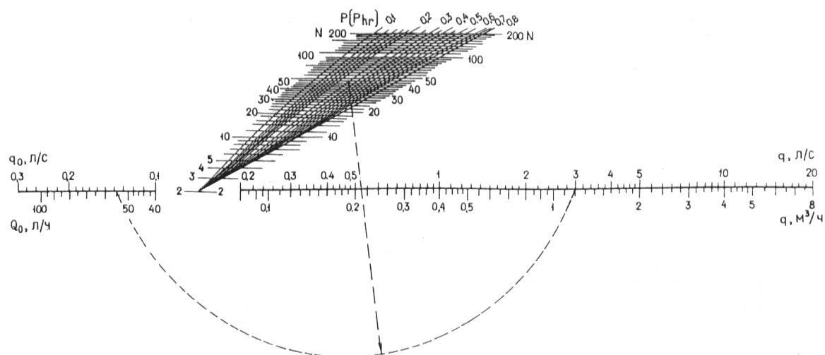
Черт.3. Номограмма для определения секундных и часовых расходов воды q при q_0 \leq 0,3 и 0,14 \text{ л/с} , N \leq 200 и P > 0,1
